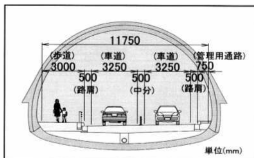
トンネル断面図
