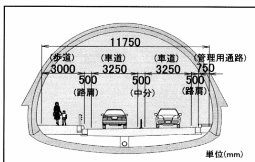
トンネル断面図
